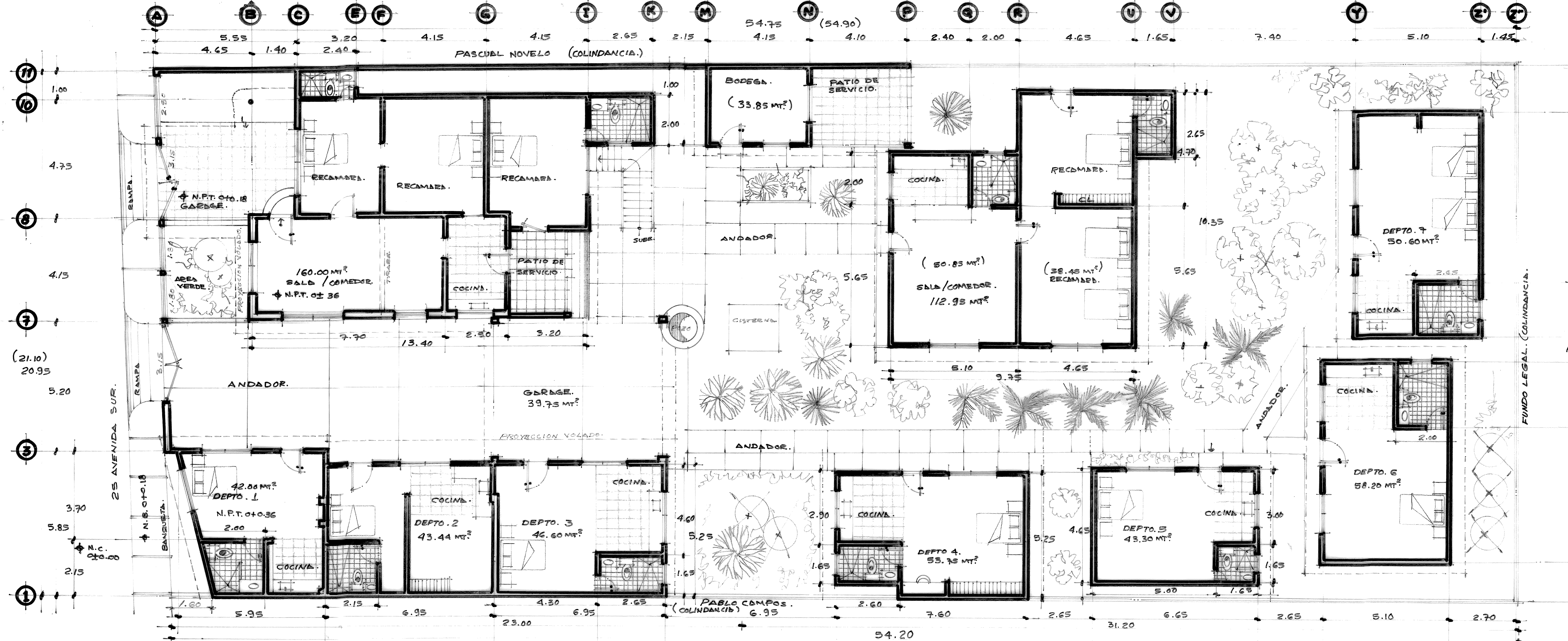
PLANTA ARQUITECTONICA BAJA. ESCALA = 1:75
