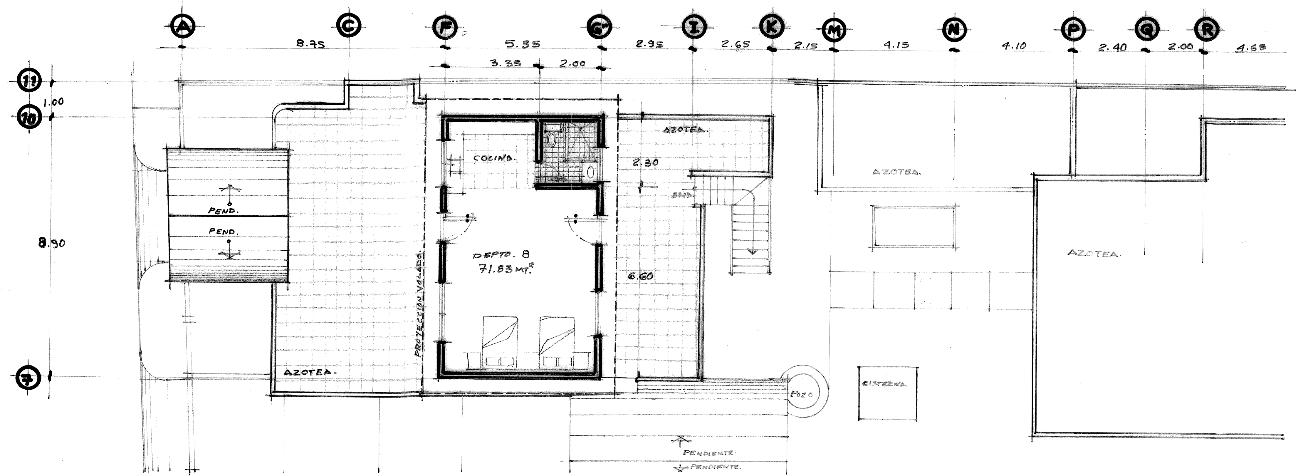
PLANTA ARQUITECTONICA ALTA. ESCALA = 1:75
